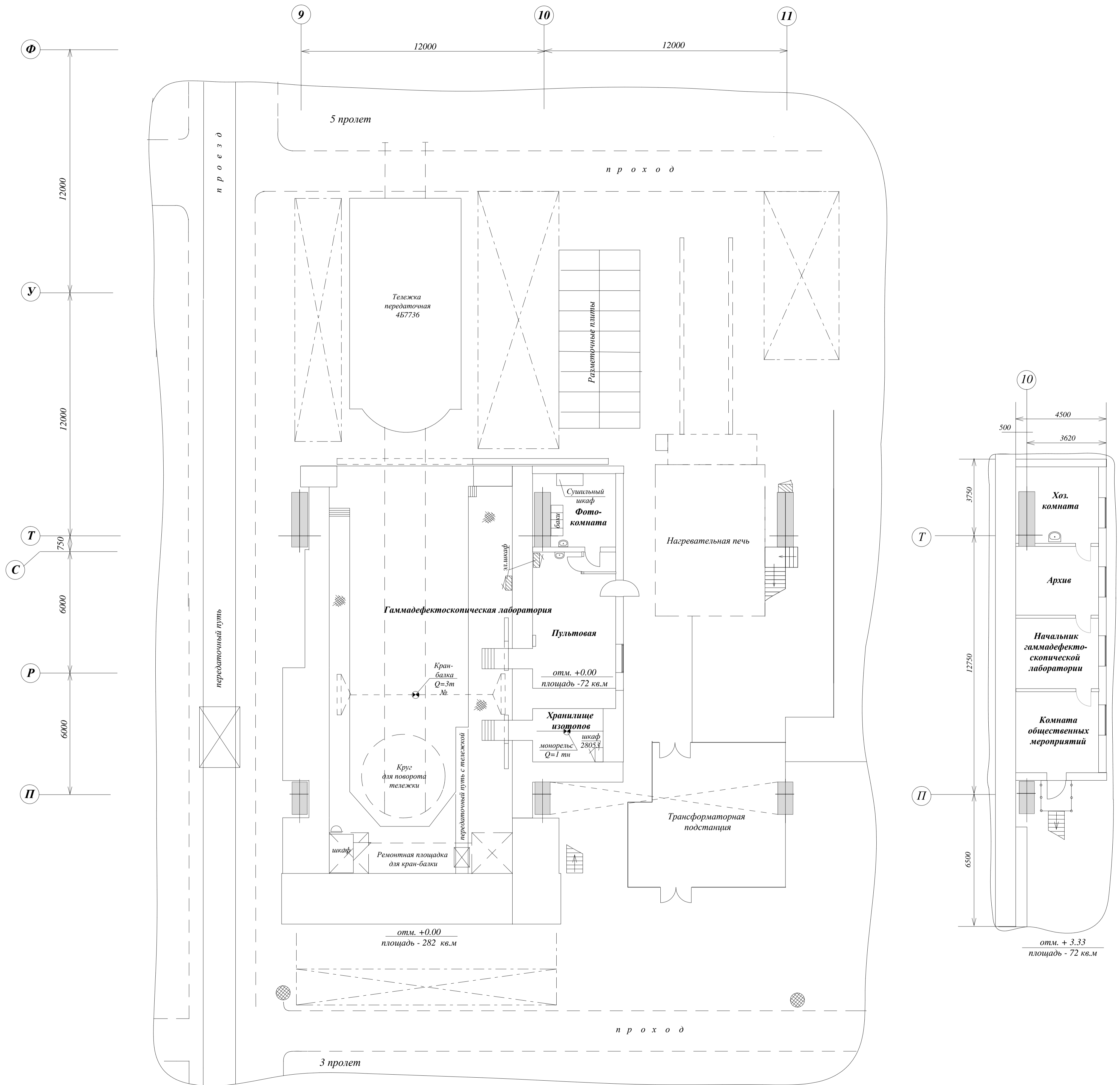
План расположения гамма-лаборатории ЦЛНМК в 4 пролете корпуса № 15
